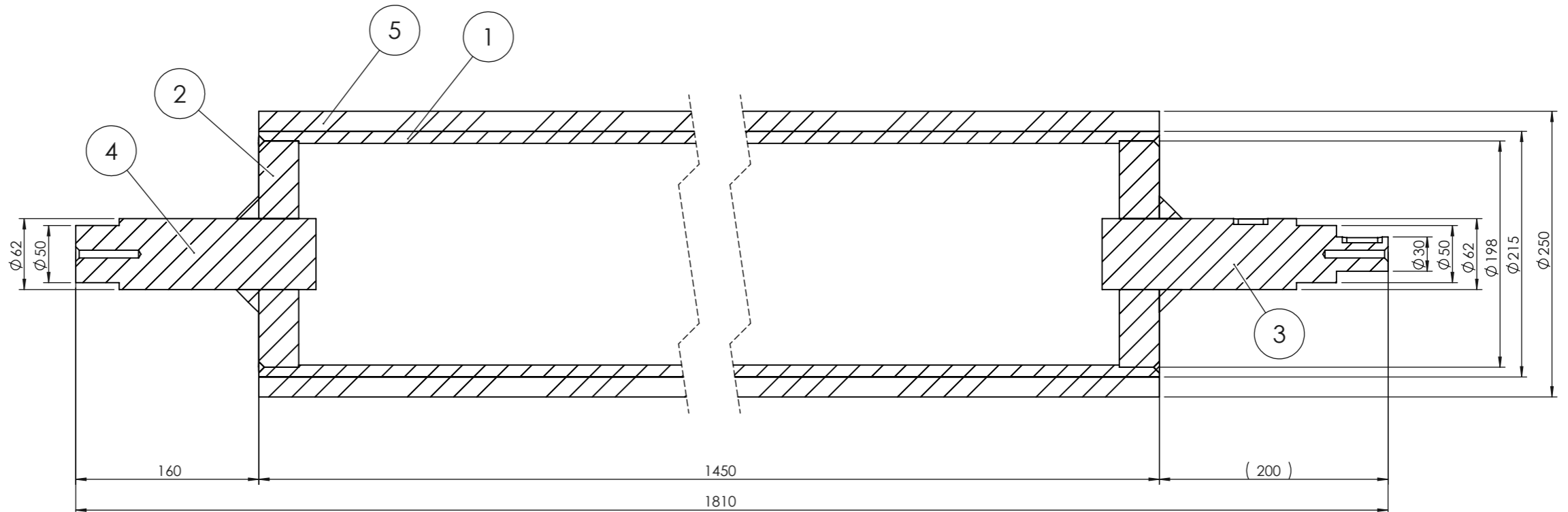
SEZIONE A-A
